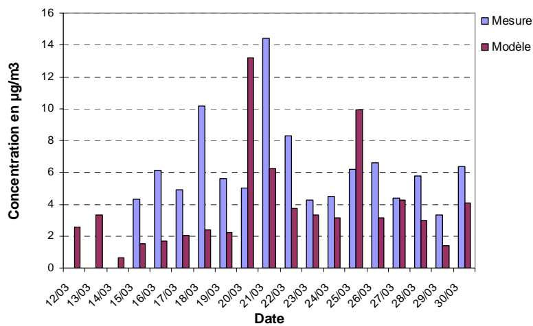
Comparaisons Mesures/Modèle - Sulfate
