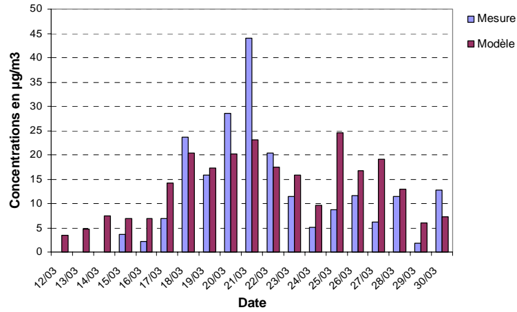
Comparaisons Mesures/Modèles - Ammonium
