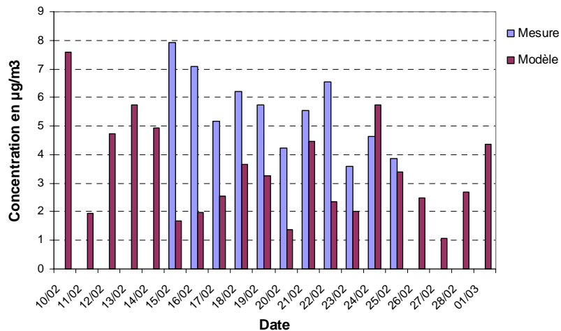
Comparaison Mesures/Modèle - Sulfate
