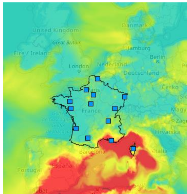
Carte de prévision PREV'AIR pour le 15/08/2021
