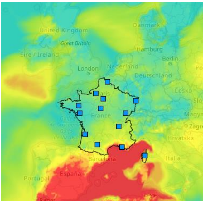
Carte de prévision PREV'AIR pour le 14/08/2021
