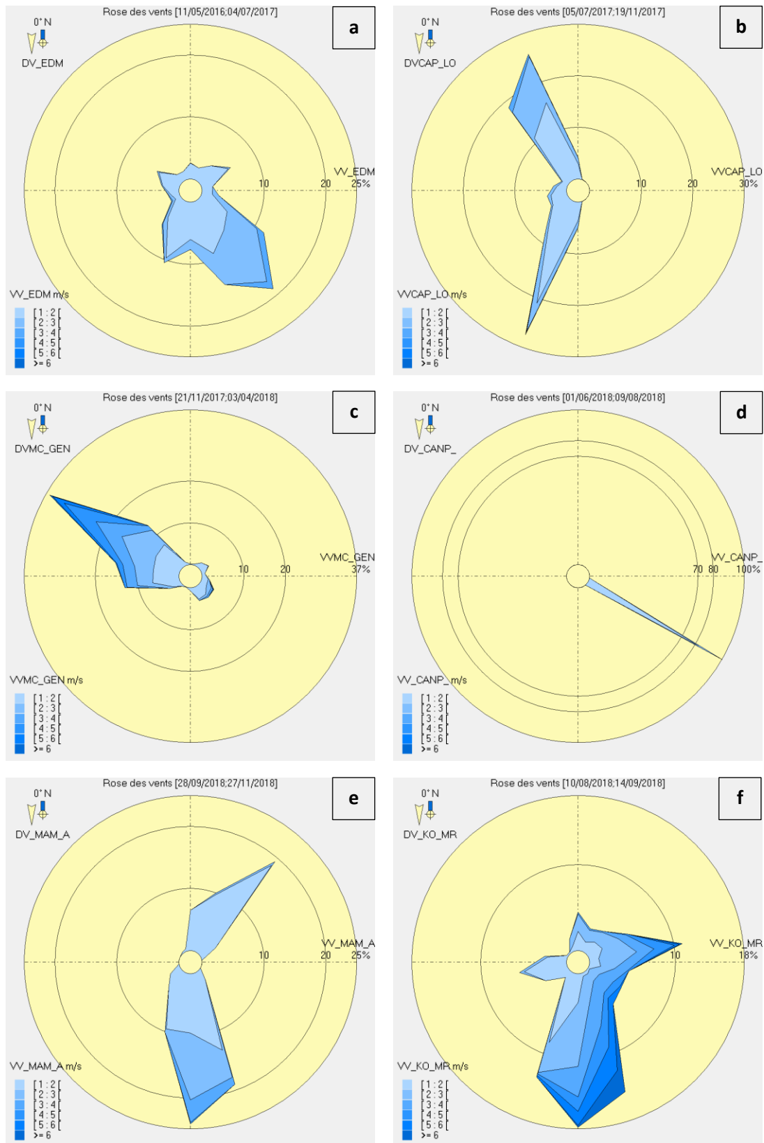
Figure 2 : Roses des vents issues des données de la station météo du laboratoire mobile (a: Kawéni ; b: Longoni; c: Pamandzi ; d: Hauts Vallons ; e: Koungou; f: Mamoudzou)
